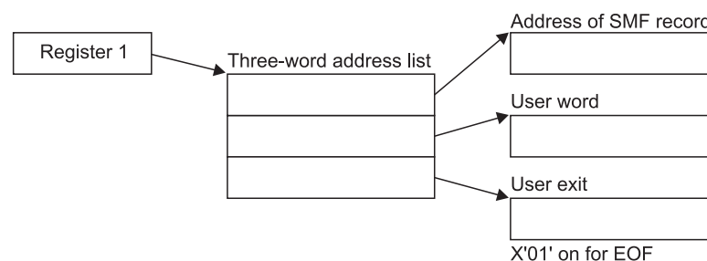
Figure 16. ERBMFPUS Input Parameter Structure
