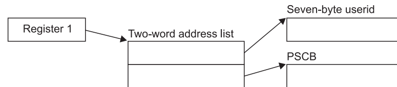
Figure 22. ERBT SOCK Input Parameter Structure
