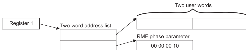
Figure 12. ERBMFRUR Input Parameter Structure
