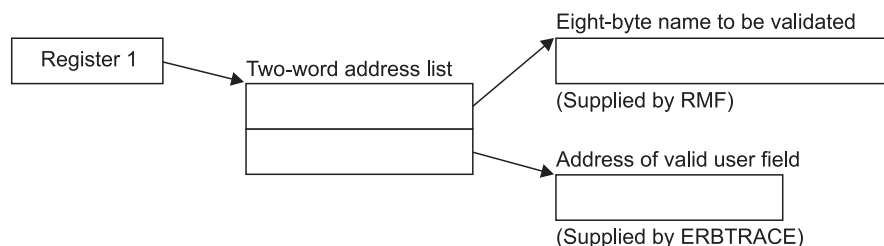
Figure 15. ERBTRACE Input Parameter Structure
