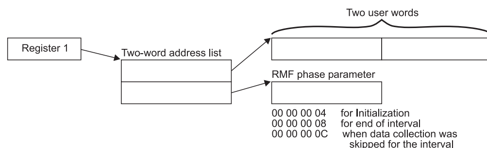
Figure 11. ERBMFDUC Input Parameter Structure
