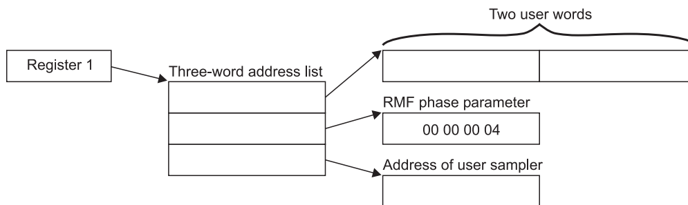
Figure 9. ERBMFIUC Input Parameter Structure
