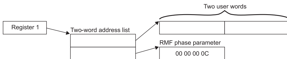
Figure 13. ERBMFTUR Input Parameter Structure
